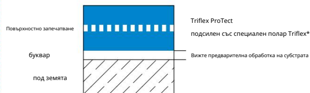
Структура на системата – детайл
