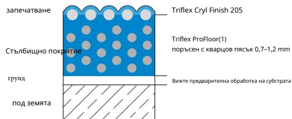
Структура на системата – детайл
